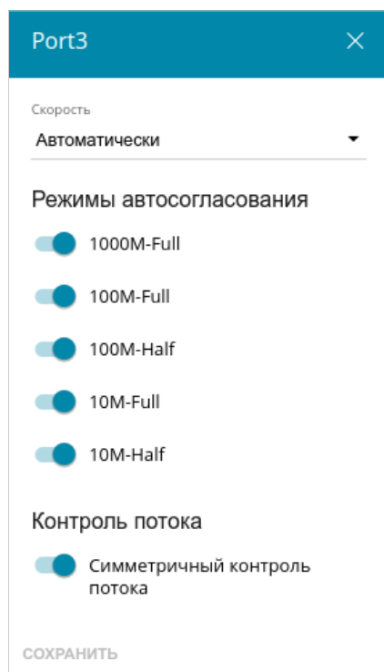
Рисунок 132. Окно изменения настроек порта межетевого экрана.
