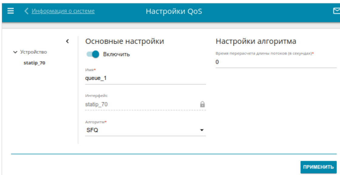
Рисунок 96. Страница QoS / Настройки QoS. Алгоритм SFQ.
