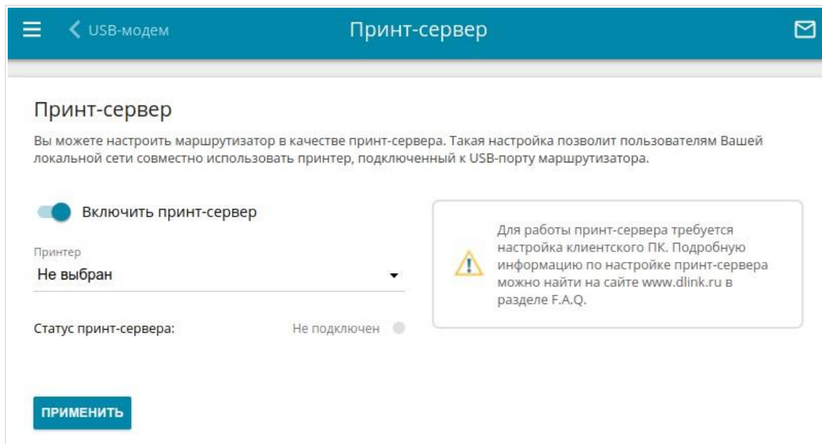
Рисунок 99. Страница Принт-сервер .
