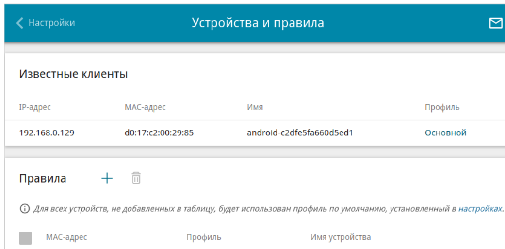
Рисунок 188. Страница SkyDNS / Устройства и правила .
