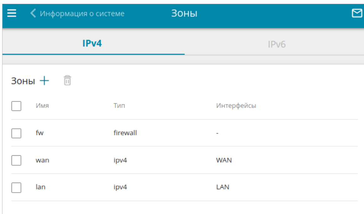
Рисунок 161. Страница Межсетевой экран / Зоны .
